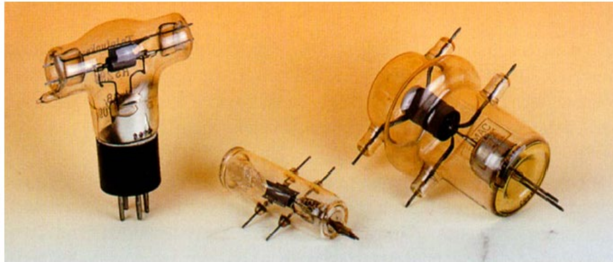
Tube à champ retardé RS296 et son circuit(Kühle 1932 at Telefunken)
