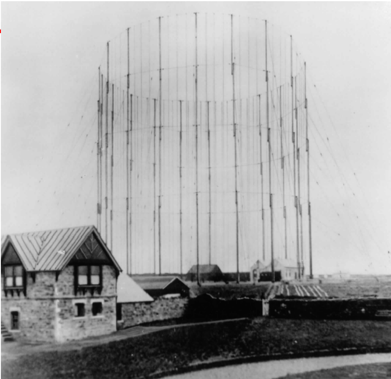
Photographie de l'antenne conique originale installée à Poldhu, Cornouaille (d'après BAE Systems Marconi Research Centre, Chelmsford, Essex )
